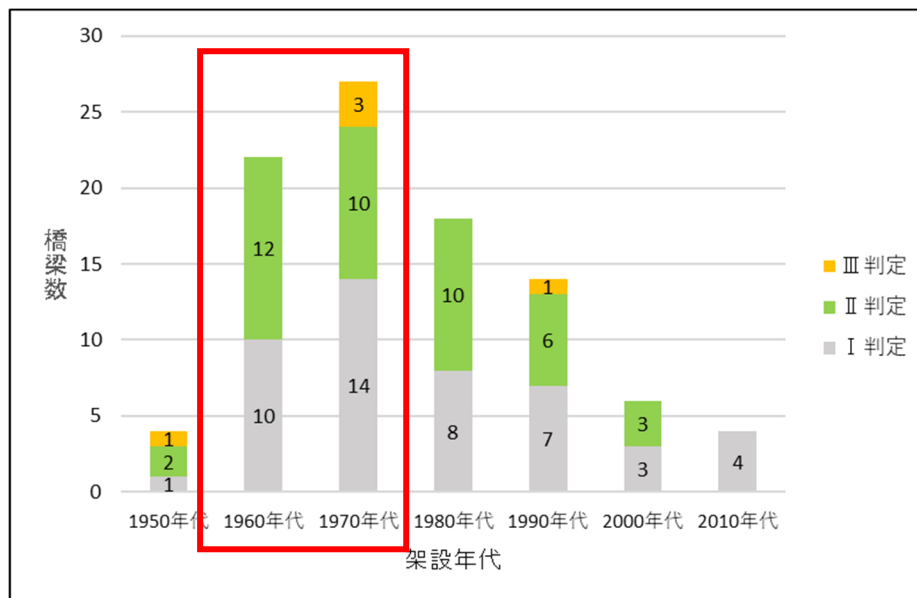
架設年代別の健全度数
