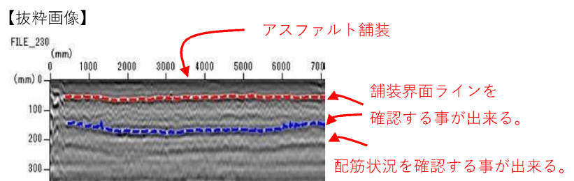
探查画像例：夫神橋
