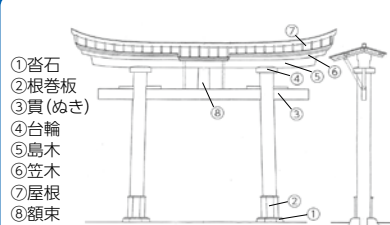
【恋渡神社一の鳥居姿図と断面図】 10数年前の修理再建時に作製。建造年代と関係工匠や区役の名が知られる貴重な明神鳥居である。
